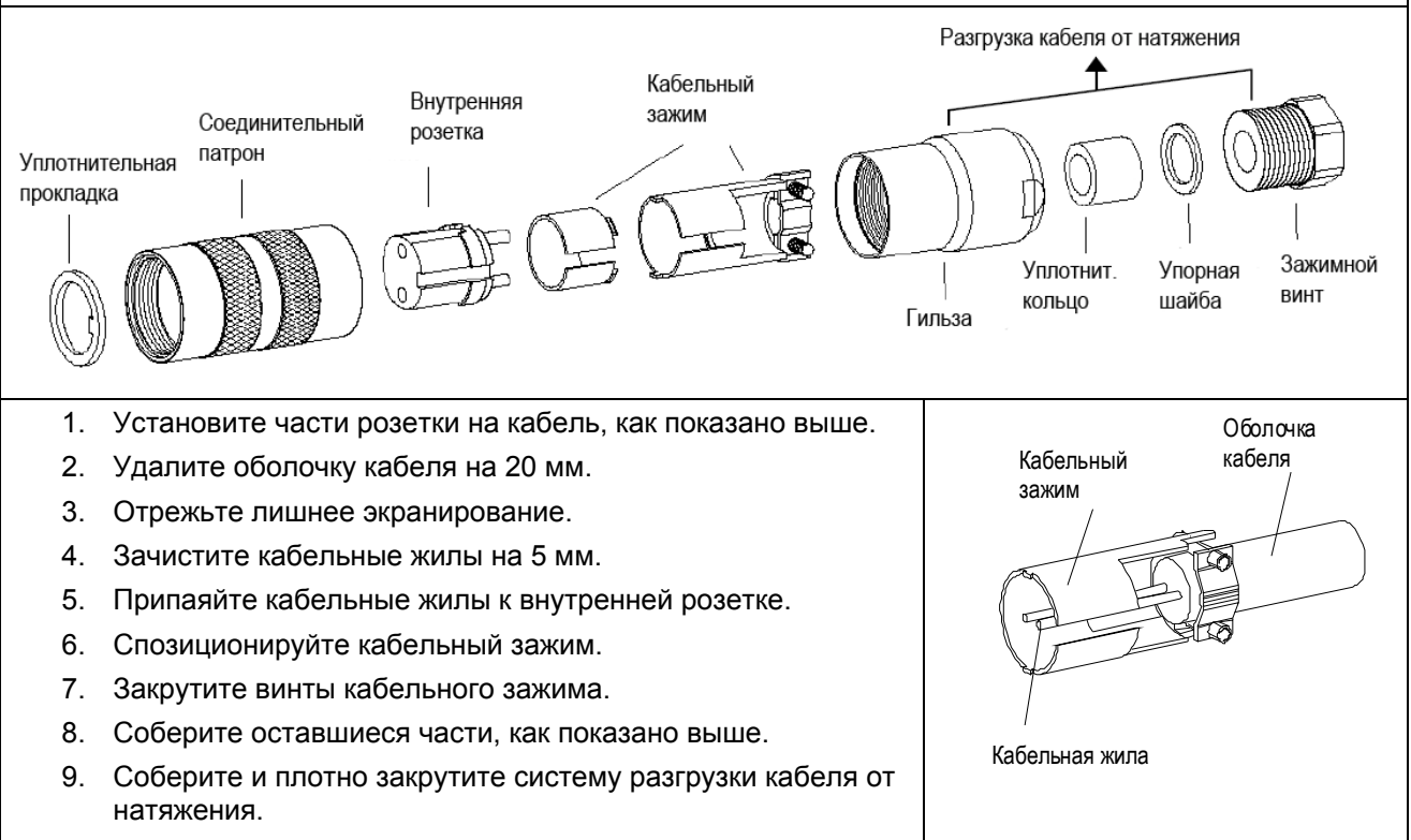
Рисунок 1: Монтаж штекера
